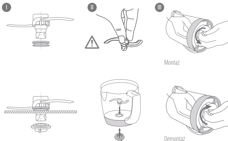
Demontaż
